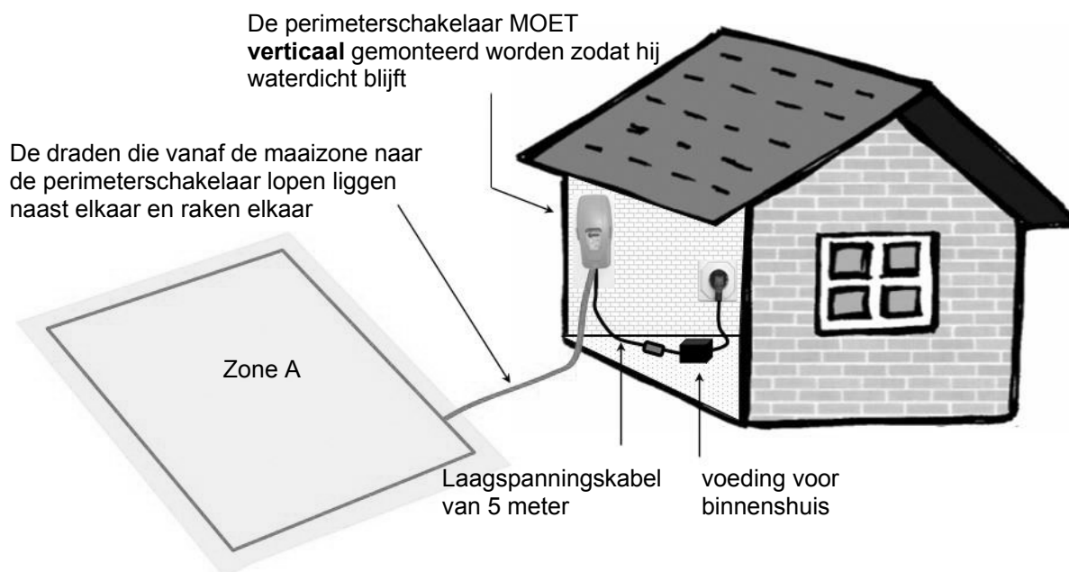
Figuur 1.2 Locatie van de perimeterschakelaar
